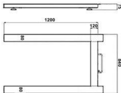
Skizze der Palettenwaage mit MaÙen
