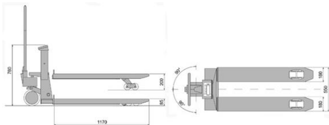
Abmessung vom Hubwagen mit interner Waage
