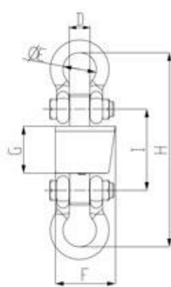
Abmessungen der Kranwaage (siehe Zeichnung)
