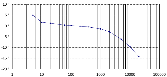
Phasenfehler Messbereich 3000 A
