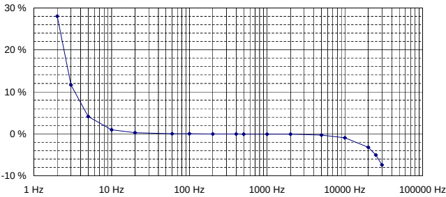
Error de magnitud rango 30 A
