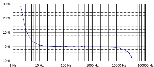
Errore d'ampiezza portata 30 A
