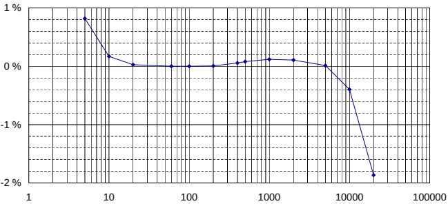
Error de magnitud rango 300 A
