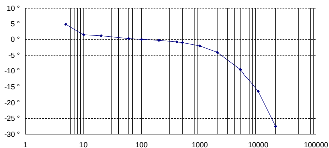
Error de fase rango 3.000 A
