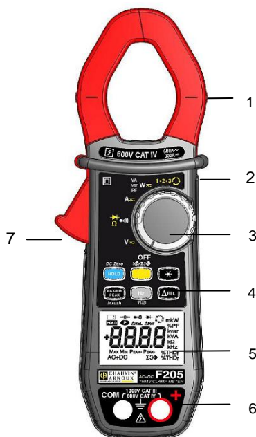
Abbildung 1 : Vielfachmesszange F205
