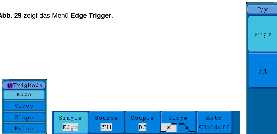
Abb. 29 Edge-Triggermenü
