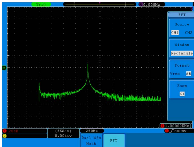
Abb. 20 Rechteck Fenster
