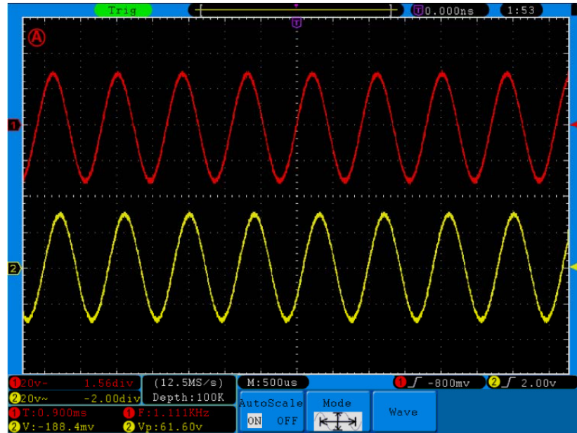
Abb. 77 Autoscale-Funktion: Mehrfachperioden-Wellenformen Horizontal-Vertikal
