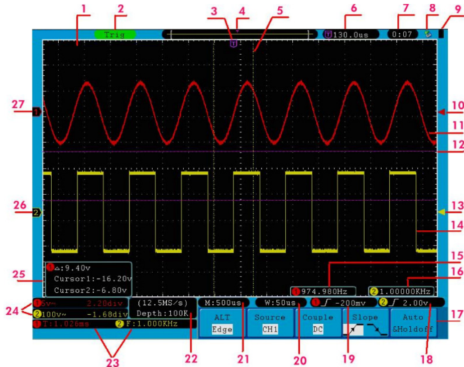
Abb. 5 Benutzeroberfläche
