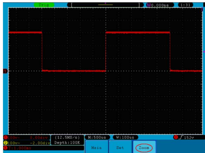
Abb. 28 Fensterausschnitt
