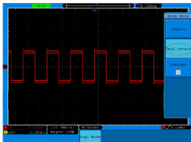
Abb. 38 Max Erkennungs-Mode, mit deren Hilfe die Spitzen der fallenden Flanke ermittelt werden können und Rauschen festgestellt wird.
