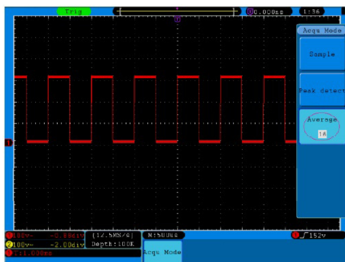
Abb. 40 die angezeigte Wellenform nachdem das Rauschen mit dem Average Mode entfernt wurde. Die Averagenummer wurde eingestellt auf 16.
