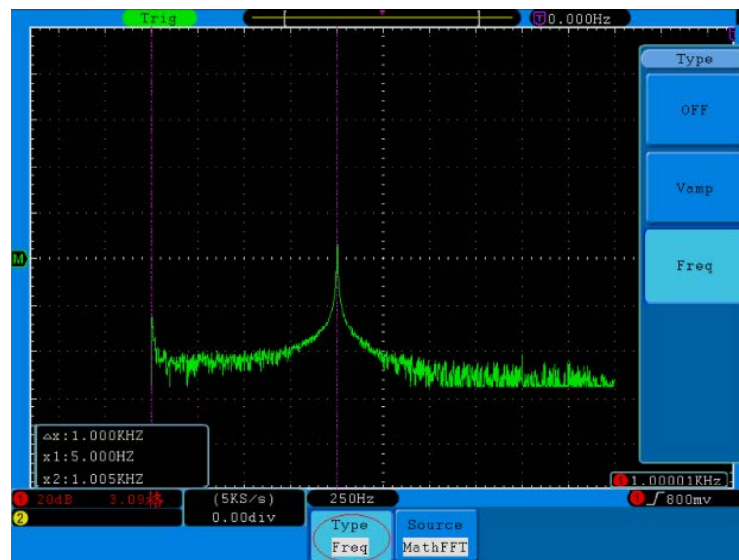
Abb. 75 Wellenform der Freq-Cursormessung
