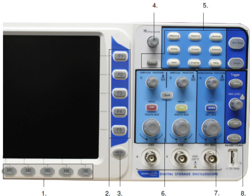
Abb. 4 Überblick über die Tasten
