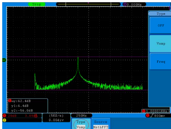
Abb. 74 Wellenform der Vamp-Cursormessung
