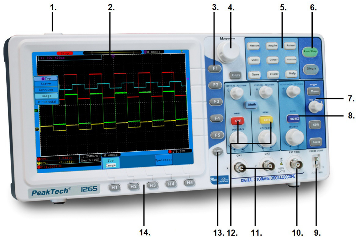
Abb. 1
