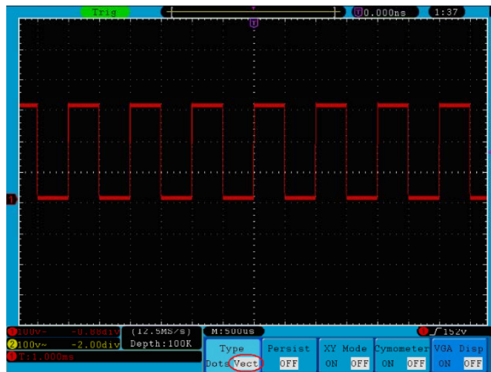
Abb. 42 Anzeige im Vektorformat
