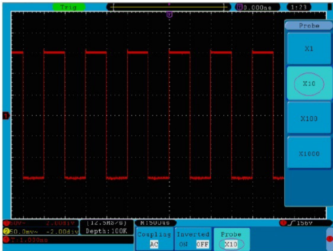
Abb. 15 Einstellen des Tastkopf-Dämpfungsfaktors
