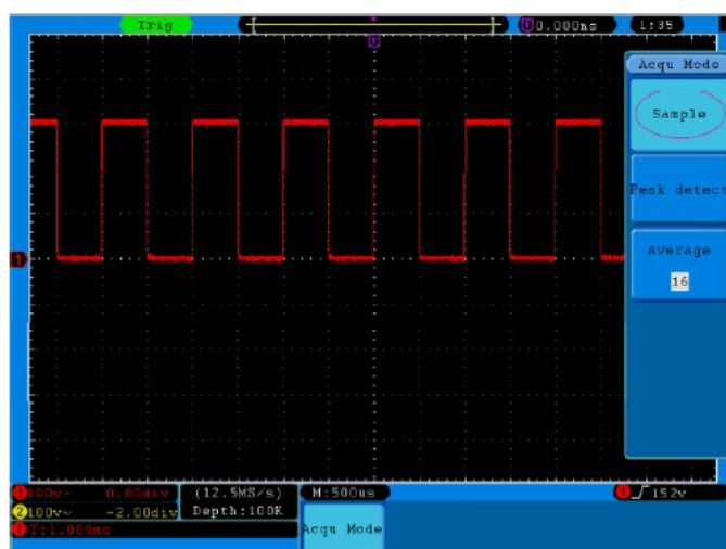
Abb. 39 übliche ACQU-Mode-Anzeige an der keine Spitzen ermittelt werden können
