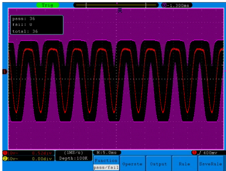
Abb.57 Pass/Fail-Prüfung
