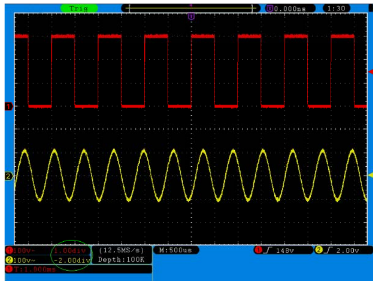
Abb. 24 Informationen zur vertikalen Position
