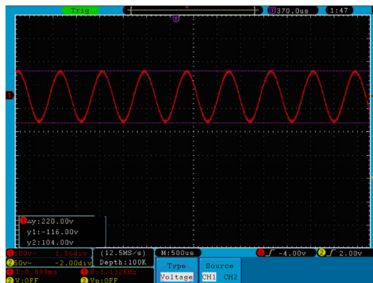
Abb. 71 Wellenform bei der Spannungsmessung mit dem Cursor
