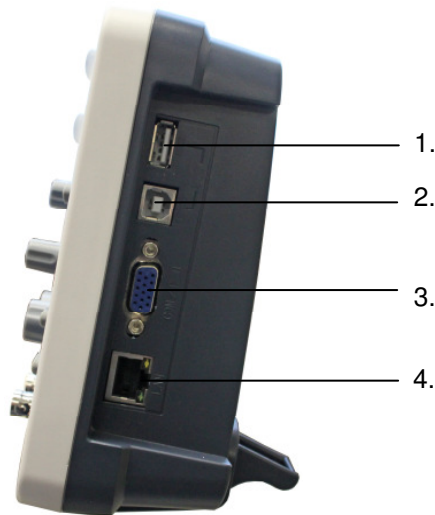
Abb. 2 Rechte Seite des Oszilloskops
