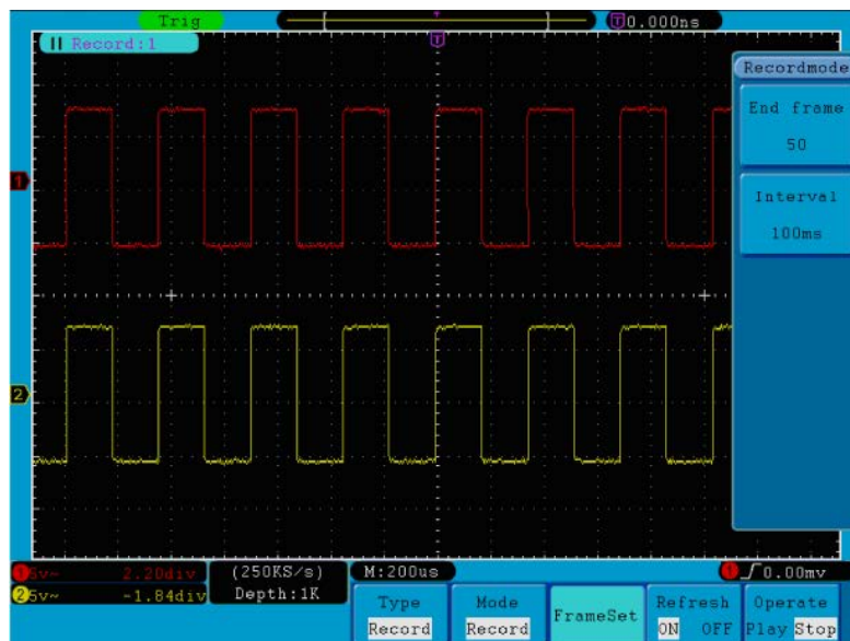
Abb. 50 Wellenform-Aufzeichnung
