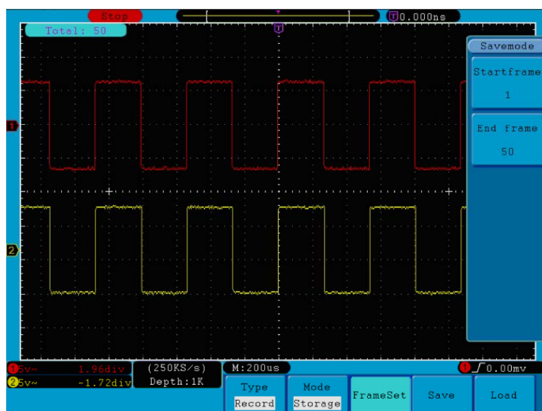
Abb.52 Wellenform-Speicherung
