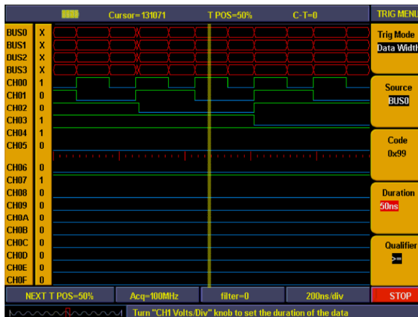
Fig. 87 Data width trigger
