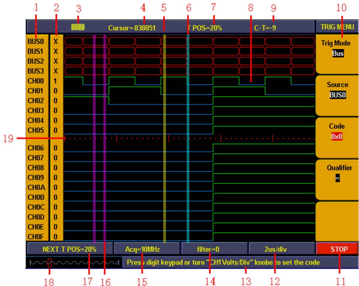
Abb. 11 Benutzerschnittstelle des Logik-Analysers
