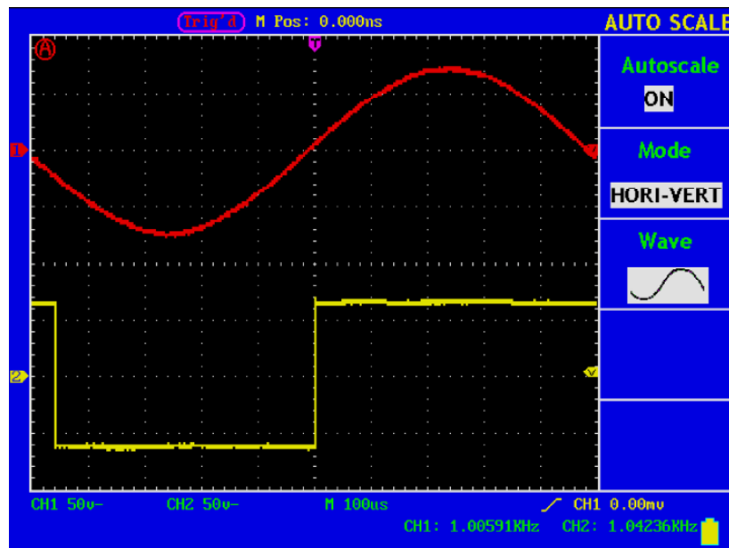
Abb. 74 Autoscale-Funktion: Einzelperiodenkurve Horizontal-Vertikal
