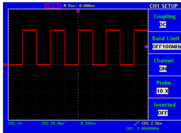
Abb. 24 Wellenform nicht invertiert
