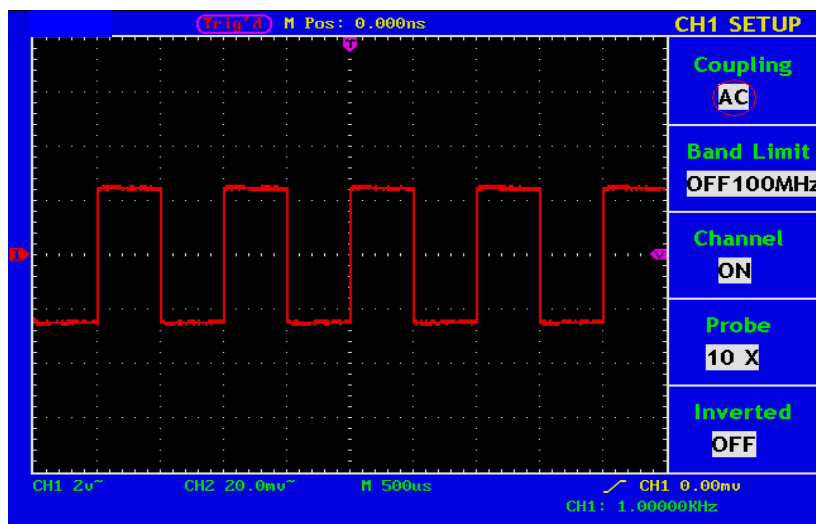
Abb. 20 AC-Kopplung Oszillogram
