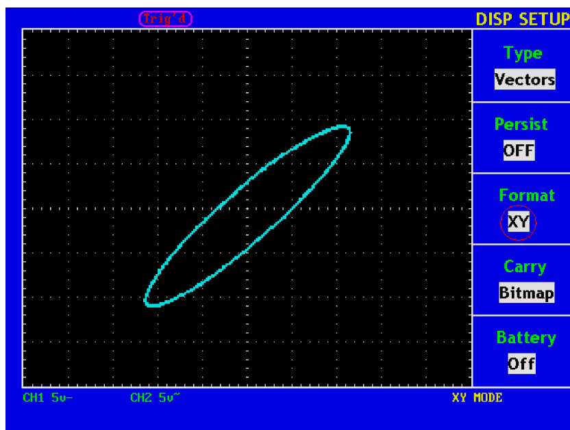
Fig. 56 XY Display Mode
