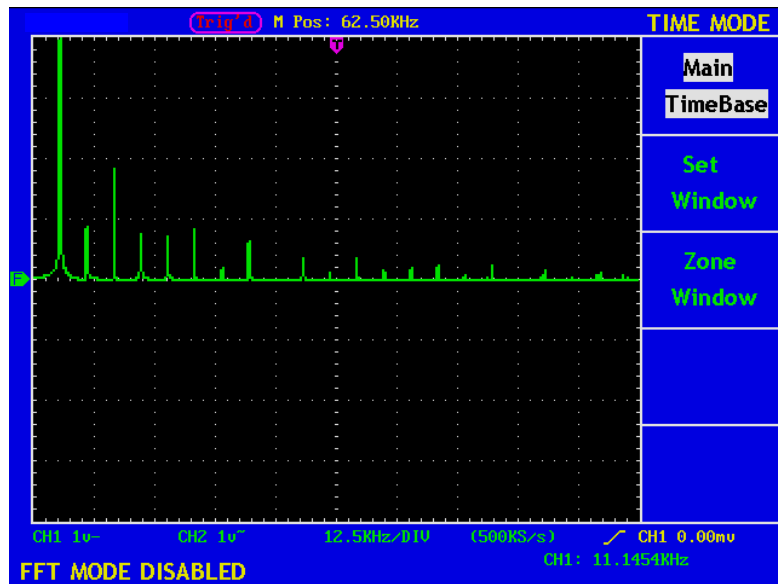
Abb. 35 Fenstereinstellungen sind im FFT-Modus deaktiviert
