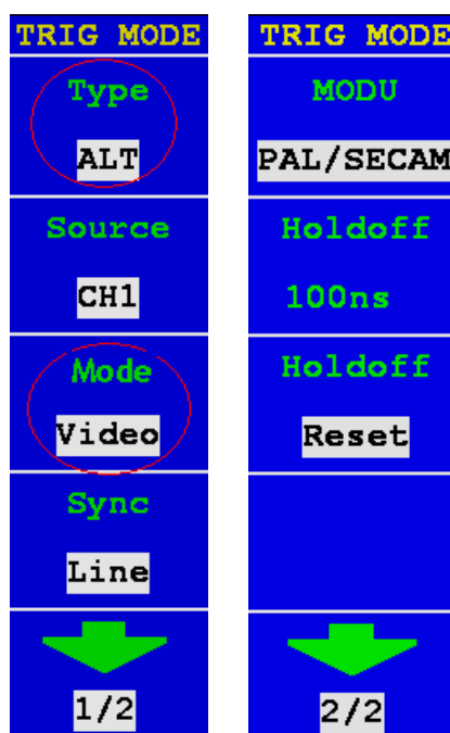
Fig. 45 Wechseltrigger (Trigger Modus: Video) Menü
