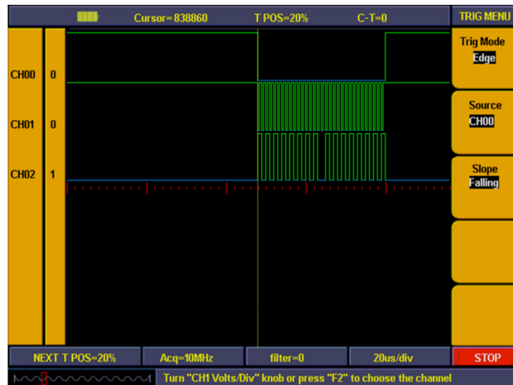
Fig. 77 Edge trigger setting
