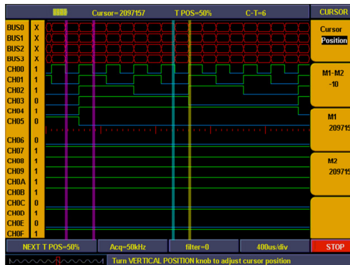
Abb. 101 Positionsmessung mit dem Cursor
