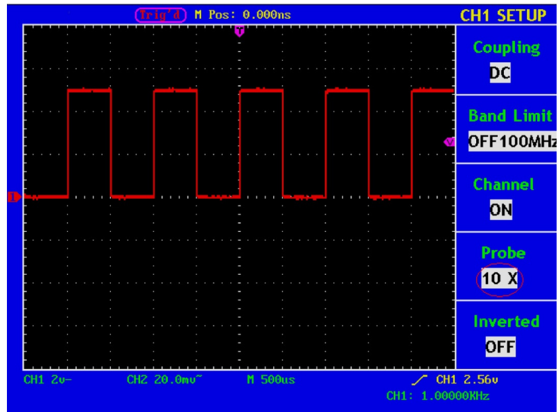
Abb. 23 Einstellen des Tastkopf-Dämpfungsfaktors
