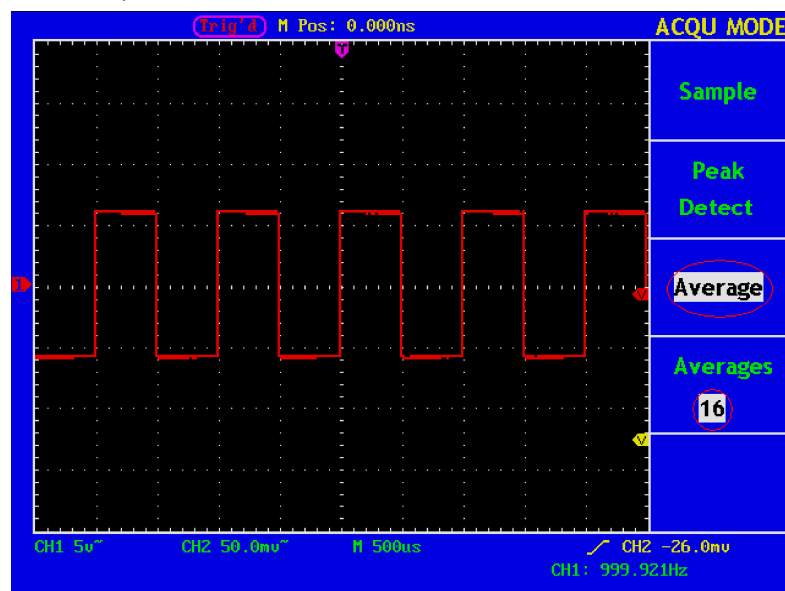
Abb. 106 Wellenform eines von Störungen befreiten Signals
