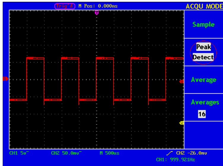
Abb. 105 Wellenform des Störimpulse enthaltenden Signals
