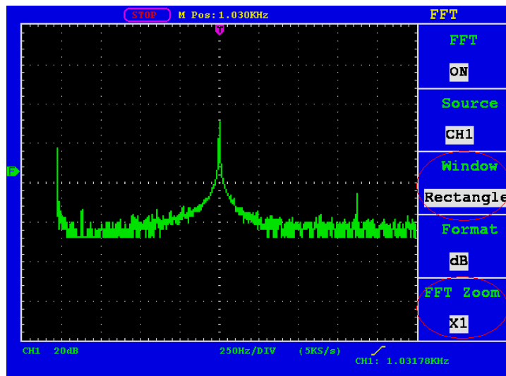
Abb. 29 Rechteck-Fenster
