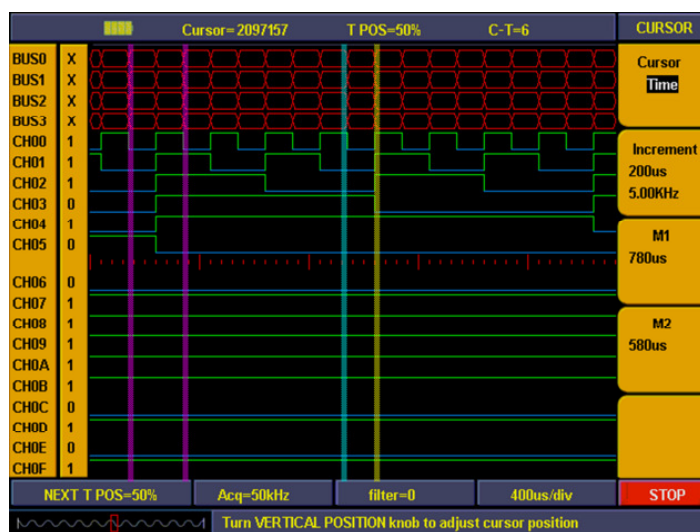
Abb. 100 Zeitmessung mit dem Cursor
