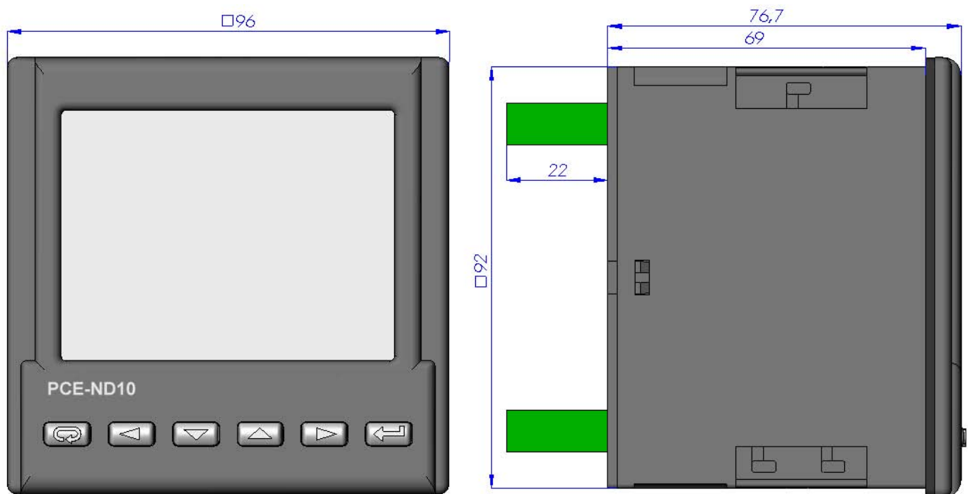
Abb. 2. Abmessungen des Messgerätes
