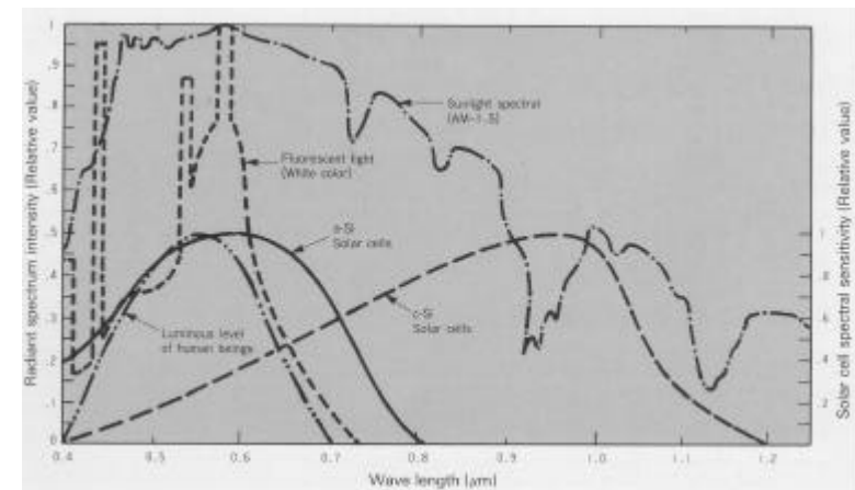
Fig. 2: Spektren verschiedener Lichtquellen und Solarzellen
