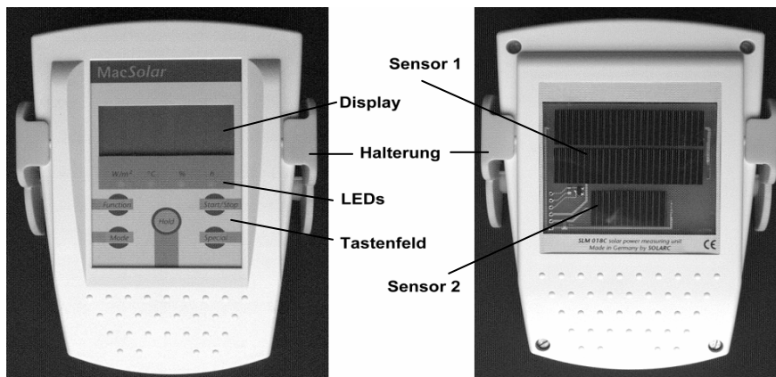
Fig. 1: Front- und Rückseite des MacSolar
