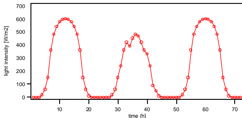
Fig. 4: Langzeitmessung im Datenloggermodus ( sto , Speicherintervall 1 h)
