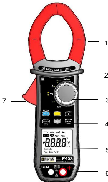
Abbildung 1 : Vielfachmesszange F403
