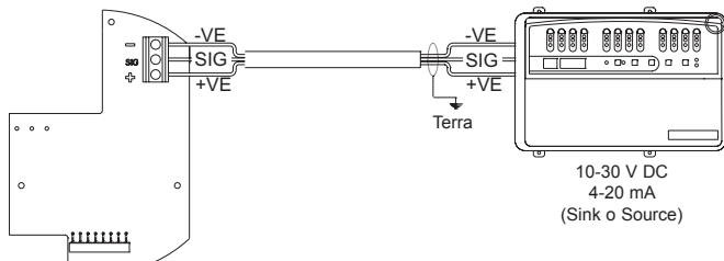
PCB per Xgard IR
